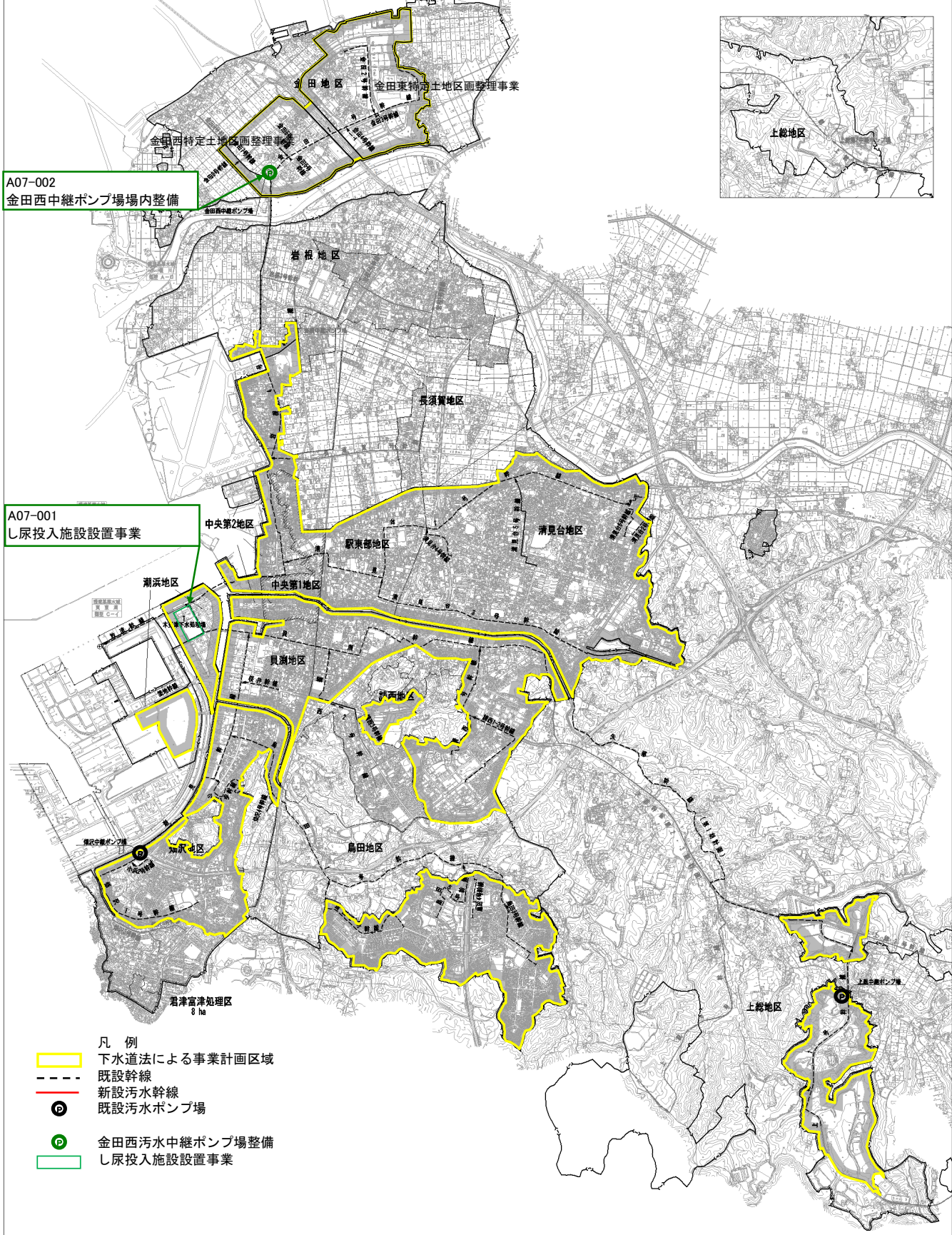
No.1木更津処理区計画図
