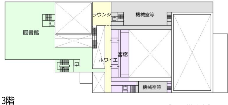
【平面構成案】
