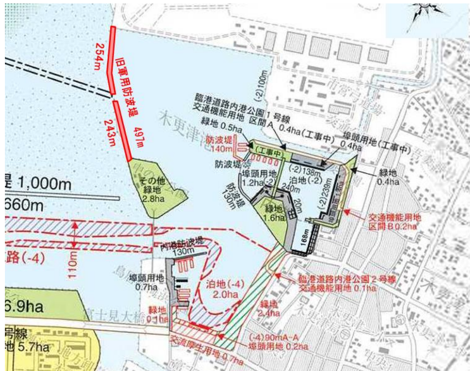
木更津港港湾計画図（平成27年2月変更）
