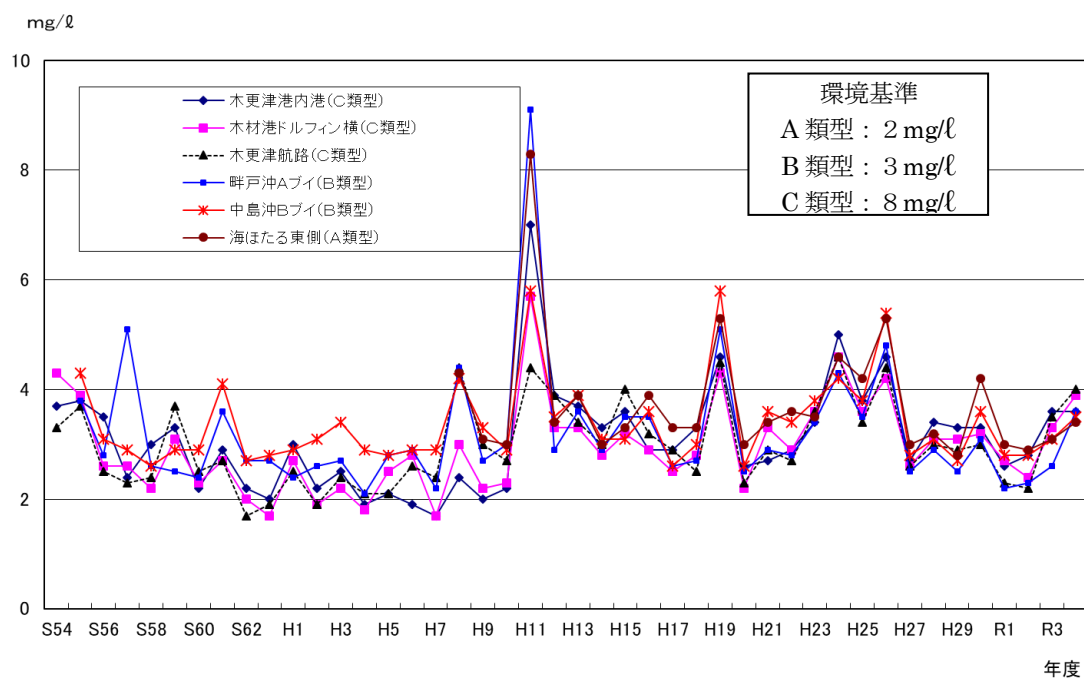
図3-2-3 海域COD（化学的酸素要求量）平均値の推移
