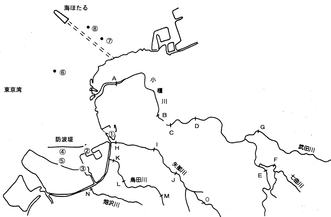
図 3 - 2 - 1 水質測定地点図
