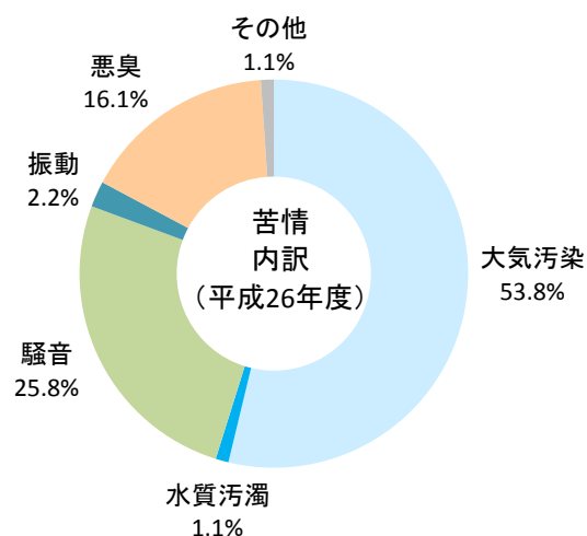
図 3-6 苦情の内訳
