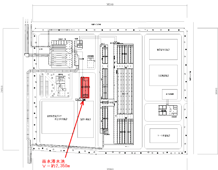
木更津下水処理場一般平面図 S=1/N
