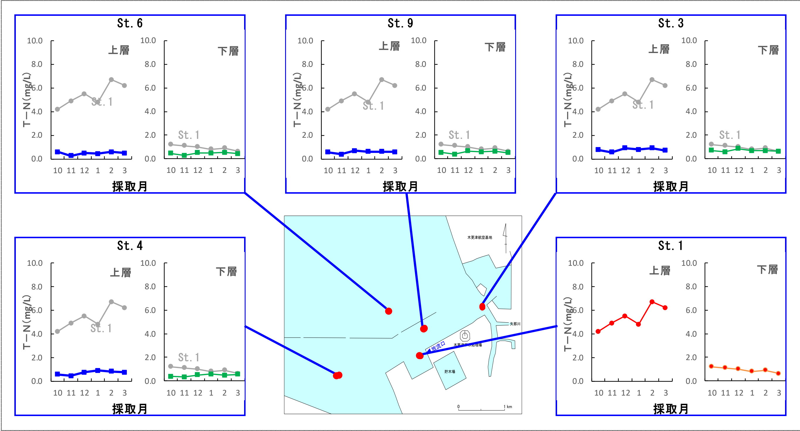
図- 5.2.2 (3) 水質の地点別経時変化（令和 5 年度）（全窒素（T-N））
