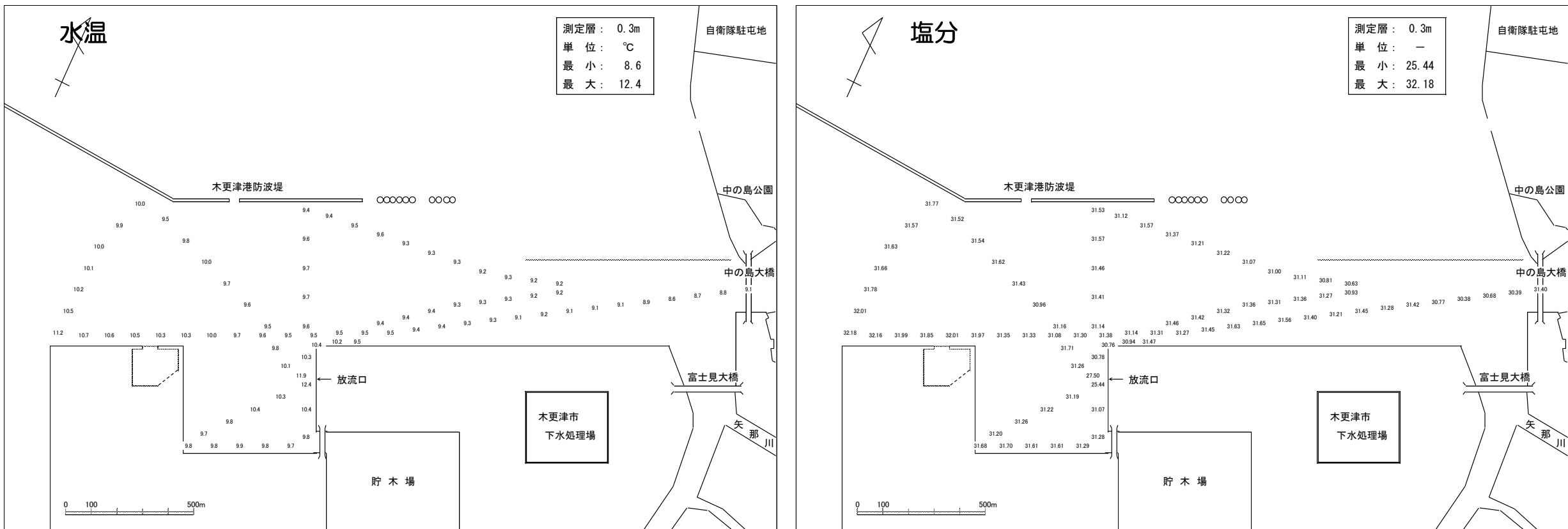
図- 5.1.1 放流口周辺海域の水温及び塩分の分布状況（海面下 0.3m：干潮時）
