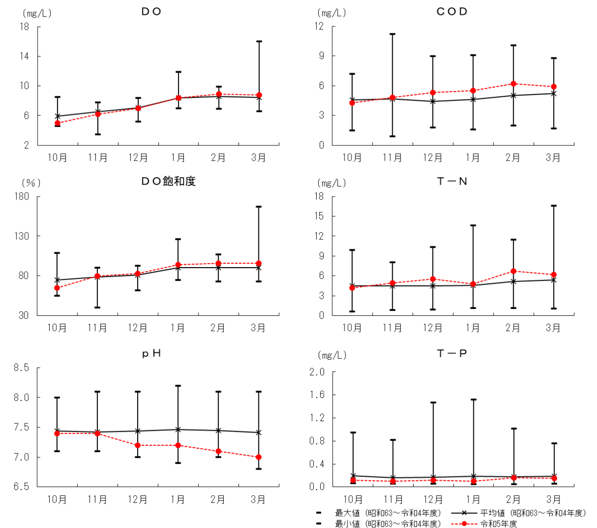
図- 5.2.1 放流口前面（St.1,上層）の水質の月別変化（昭和63年度～令和5年度）
