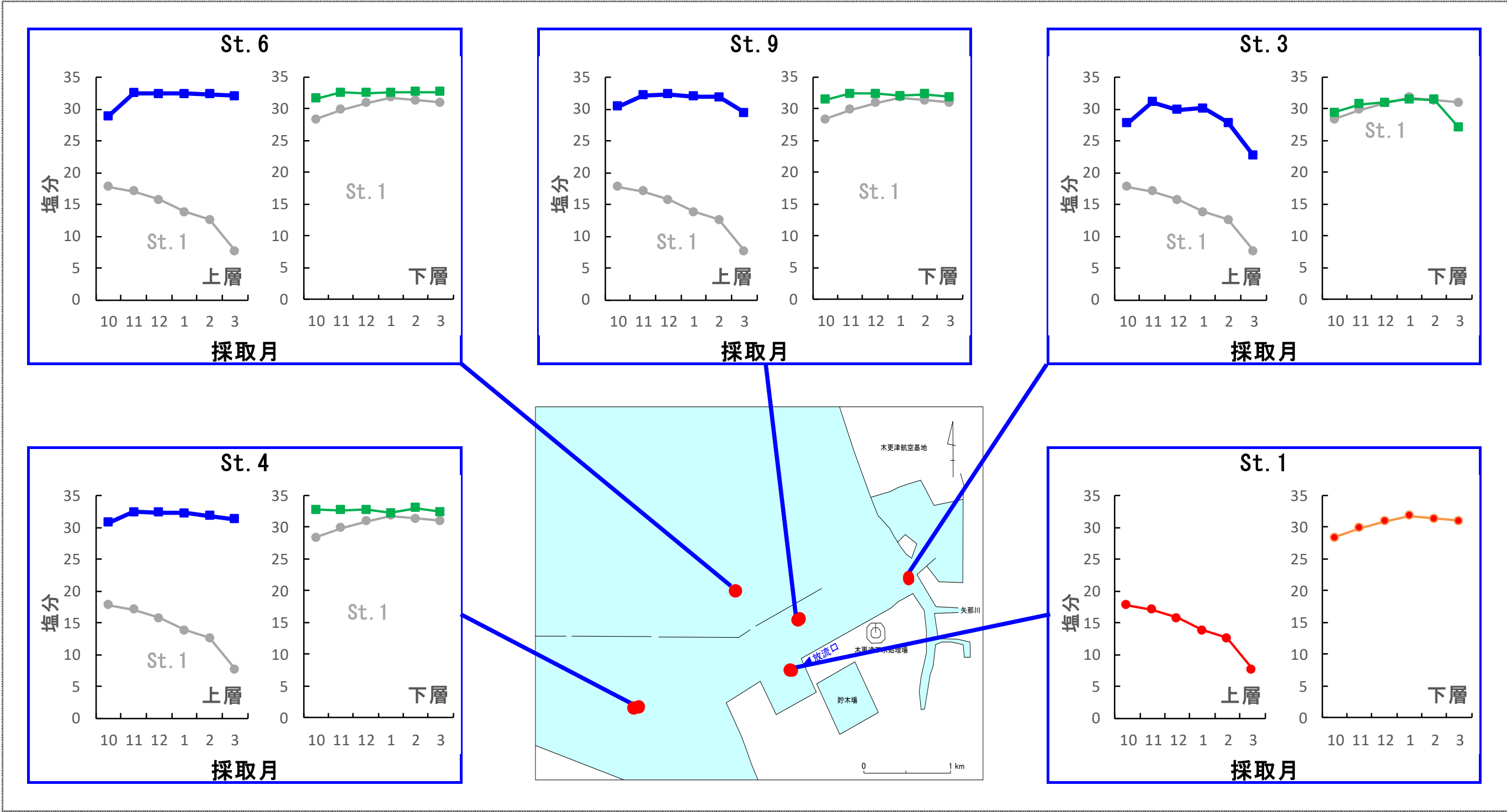
図- 5.2.2 (1) 水質の地点別経時変化 (令和 5 年度) (塩分)
