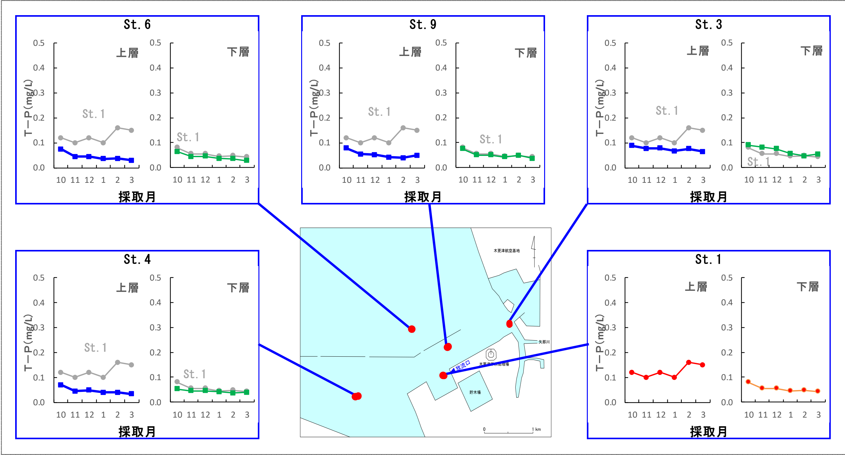
図- 5.2.2 (4) 水質の地点別経時変化（令和 5 年度）（全リン（T-P））
