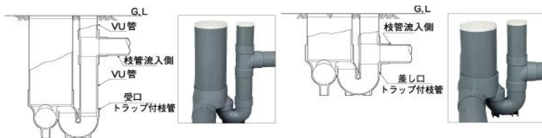
小口径のトラップ付き枳（掃除口あり）
