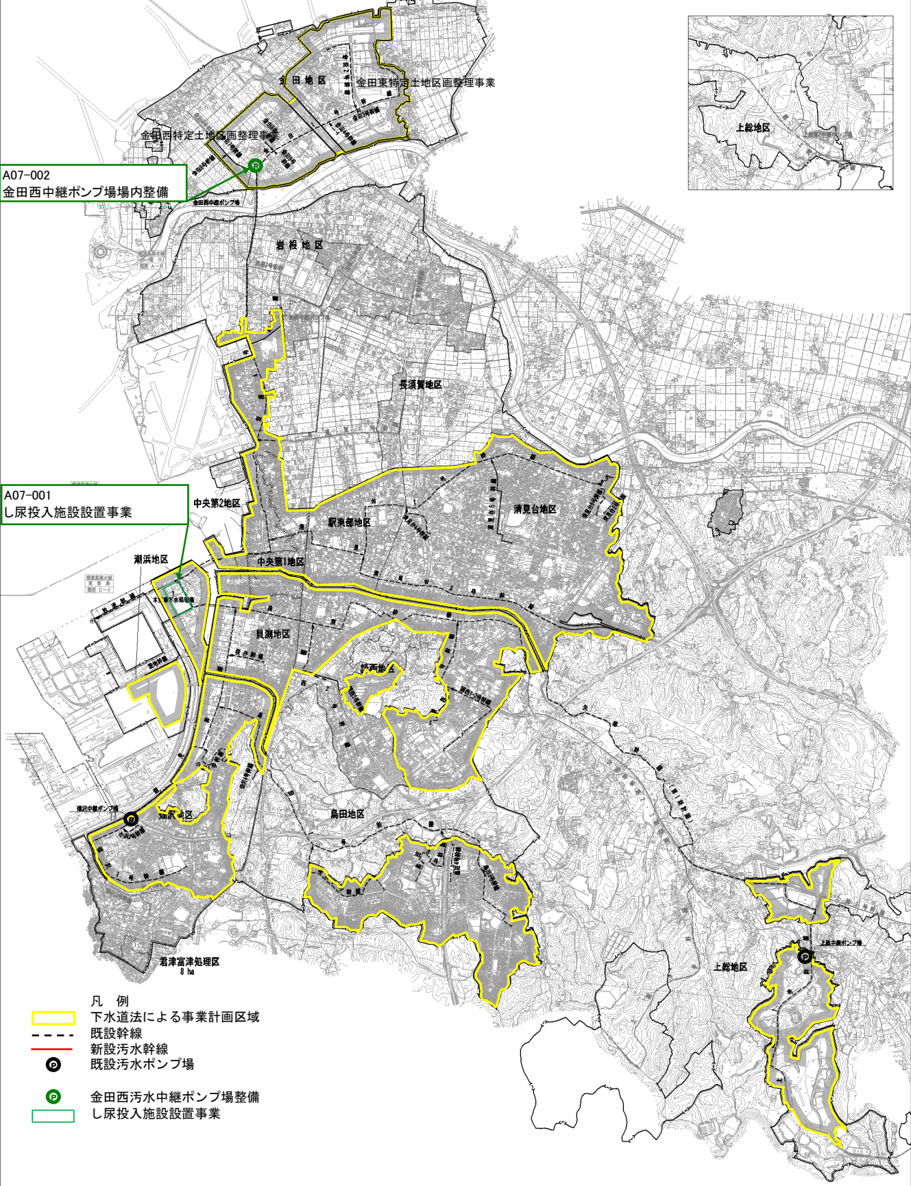
No.1木更津処理区計画図
