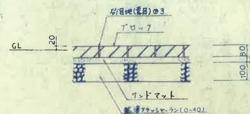
歩道部詳細図 s=1/10 (インターロッキングブロック)
