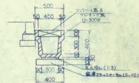
側溝詳細図 s=1/20
