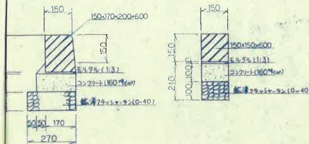
縁石詳細図 s=1/10
