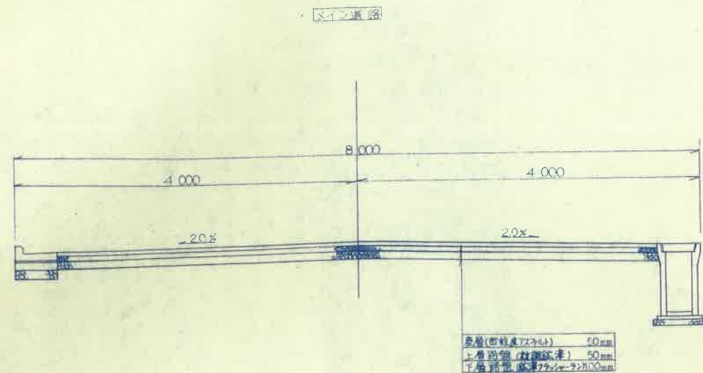
管理用道路
