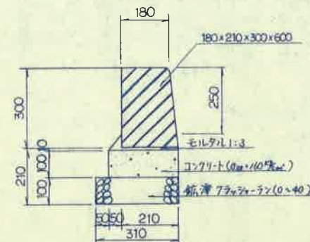
縁石詳細図 s=1/10
