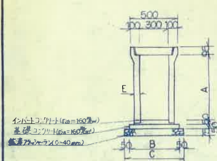
側溝敷設標準断面図 (勾配可変側溝) s=1/20
