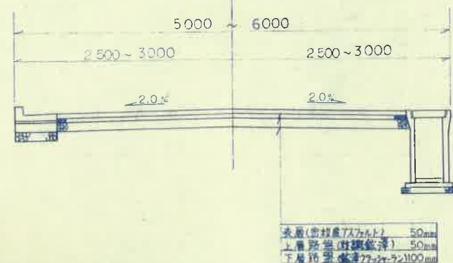
側溝敷設標準断面図 (勾配可変側溝) s=1/20
