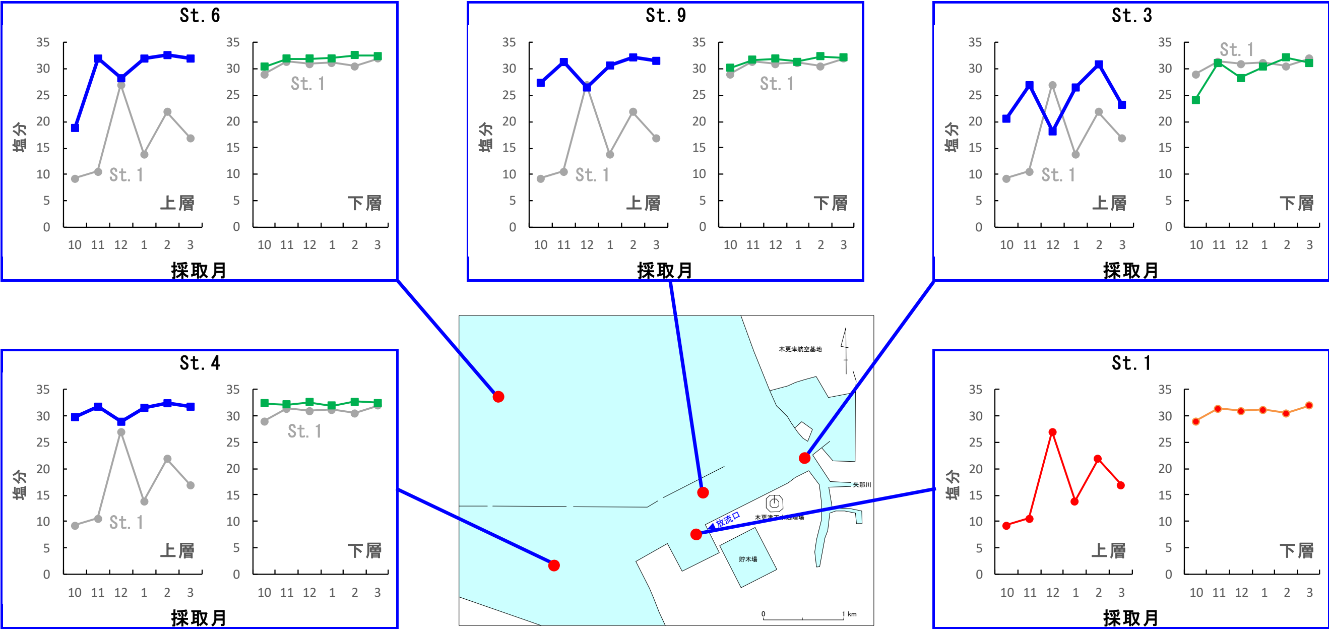
図- 5.2.2 (1) 水質の地点別経時変化（令和 3 年度）（塩分）
