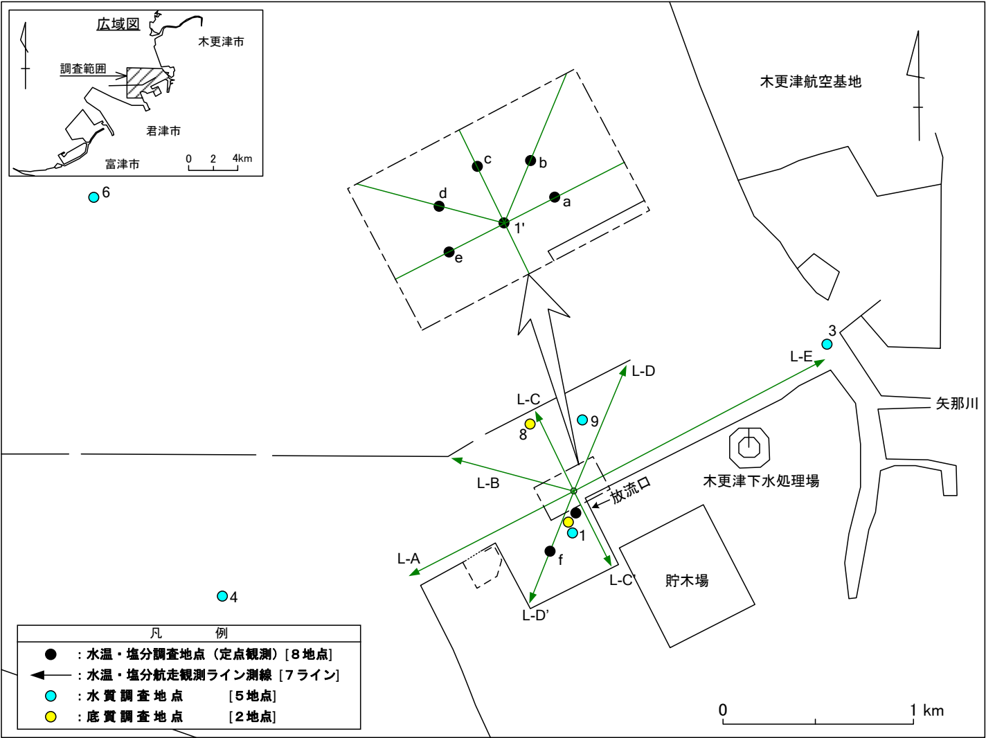
図- 3.1.1 調査地点位置
