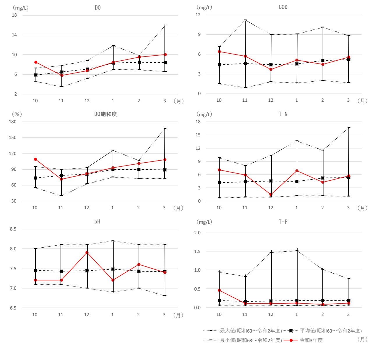
図- 5.2.1 放流口前面（St.1,上層）の水質の月別変化（昭和 63 年度～令和 3 年度）
