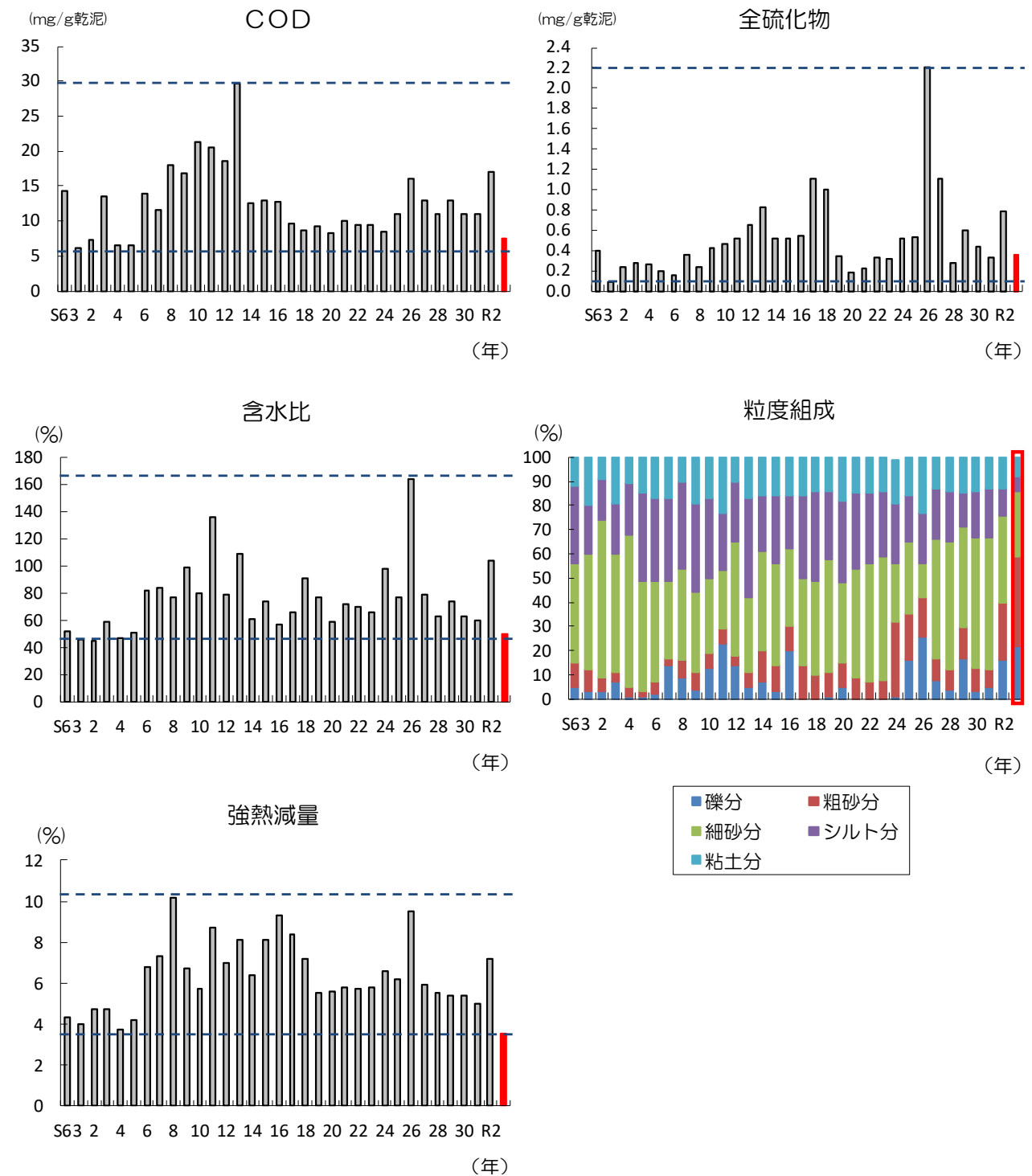
図- 5.3.2 放流口前面（St.1）の底質の経年変化（昭和 63 年度～令和 3 年度）
