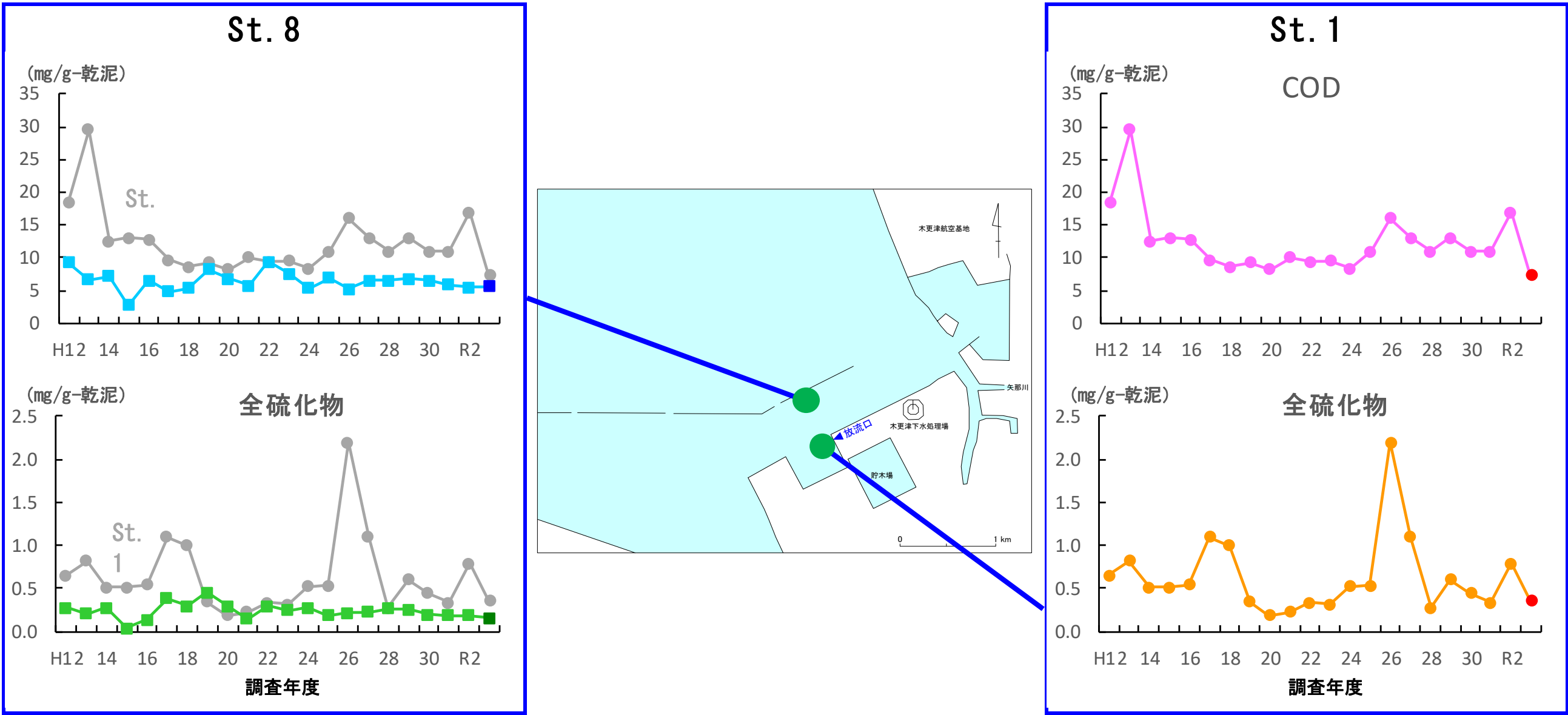
図- 5.3.3 底質（COD、全硫化物）の経年変化（平成 12 年度～令和 3 年度）
