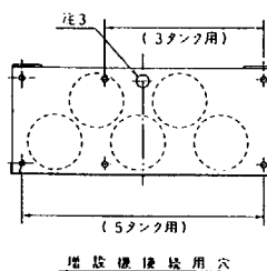
注1) 信号線（フロートスイッチ）、電源（ＡＣ100Ｖ）及び通水配管用入口：：埋設配線の場合 注2) 信号線（フロートスイッチ）、電源（ＡＣ100Ｖ）及び配通配管用入口：：露出配線の場合 注3) 信号線（フロートスイッチ）及び通水配管用入口：：増設機接続の場合
