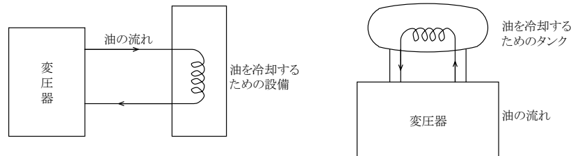
第3-12-1図 変圧器油を冷却するための附随設備
