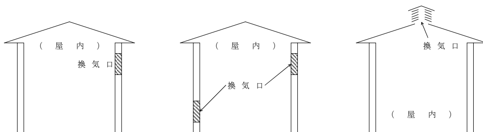
第3-1-7図 自然換気設備の例
