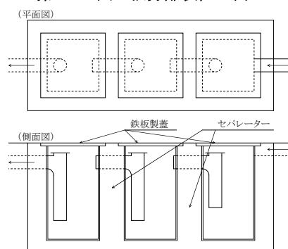
第3-1-5図 油分離装置の例
