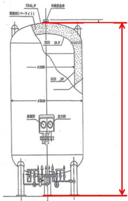
第3-9-49図 液化水素の貯槽の高さ
