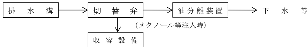
第3-9-55図 メタノール等の専用タンクの注入口及びメタノール等以外の専用 タンクの注入口の周囲に排水溝を設ける場合の例
