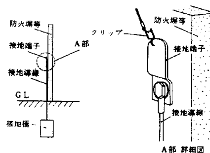
第3-3-3図 接地電極の例
