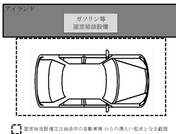
第3-9-45図 漏えい起点となる範囲
