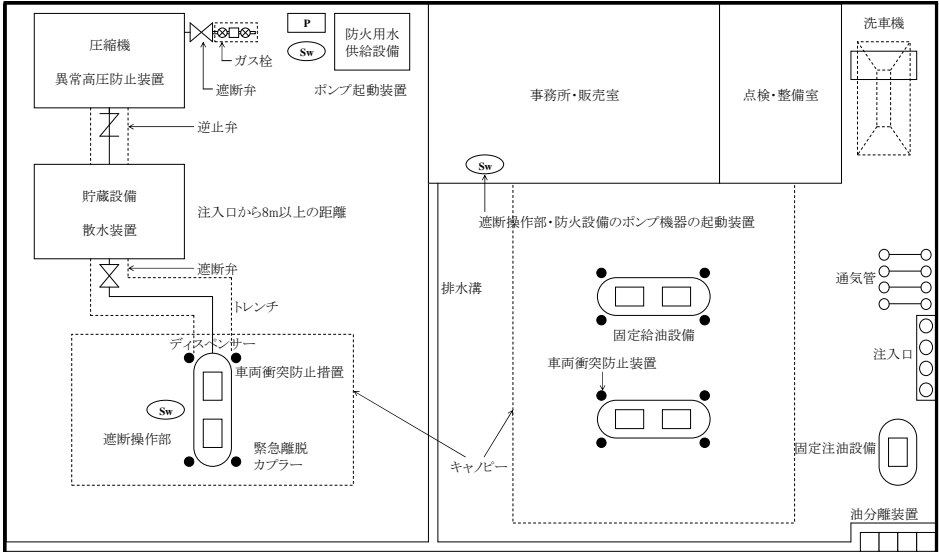
第3-9-35図 圧縮天然ガス充填設備設置給油取扱所のモデル図
