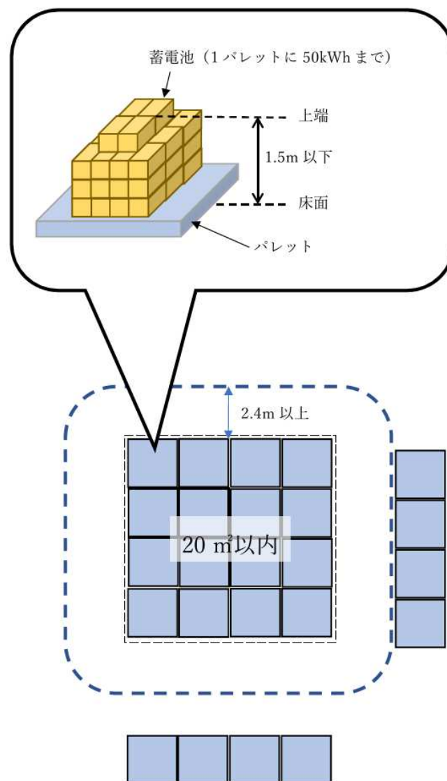
第3-2-2図 危規則第16条の2の8第2項第5号ハによる貯蔵方法の例
