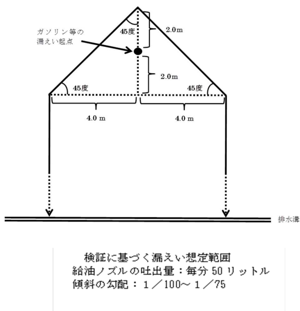
第3-9-46図 検証に基づく漏えい想定範囲
