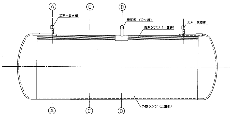
第3-5-12図 (その2) 鋼製二重殻タンクのエア一抜き部断面詳細
