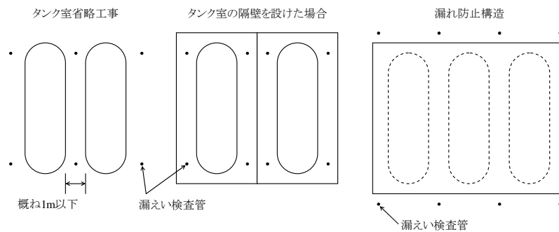
第3-5-5図 漏洩検査管の設置例
