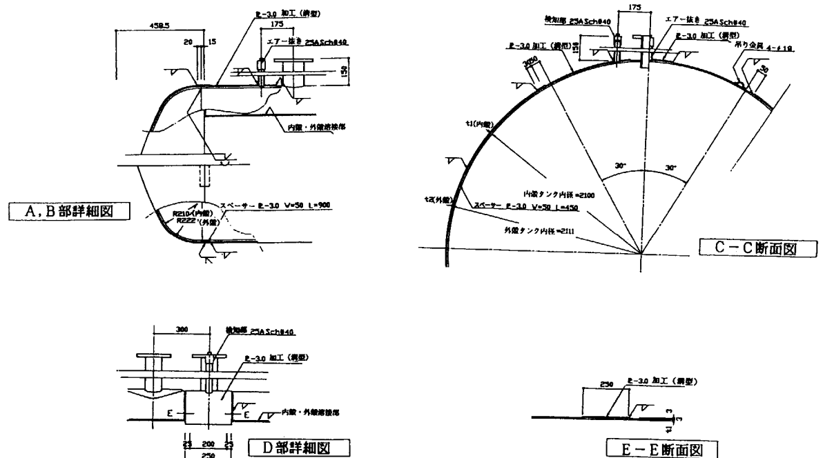
第3-5-13図 (その2の2) 鋼製二重殻タンク各部の例 (10kL 内径: 2100)
