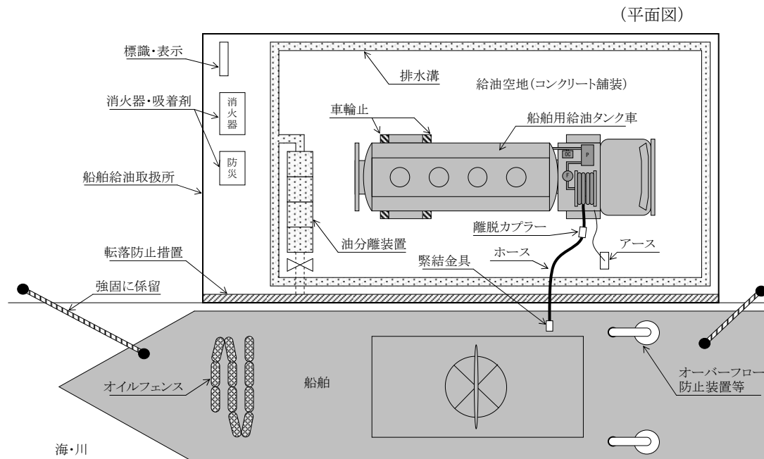
第3-9-34図 船舶給油取扱所配置例
