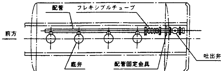
第3-7-33図 緩衝継手による底弁に直接衝撃が加わらない措置
