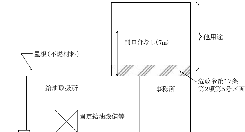
第3-9-30図 耐火構造としない屋根の例
