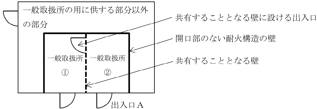
第3-12-6-2図 一般取扱所を隣接させて設置する場合の例
