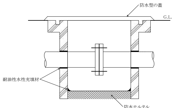
第3-1-22図 点検箱の例
