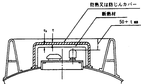
③ 防熱又は防じんカバーの間に断熱材が張り付けられているもの
