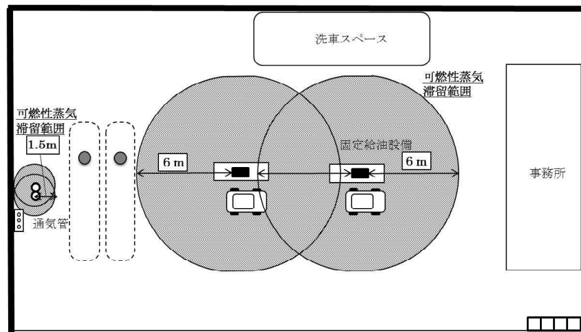
図4 給油取扱所（平面図）
