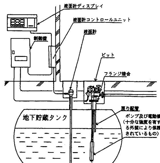
第3-5-3図 油中ポンプ設備の設置例
