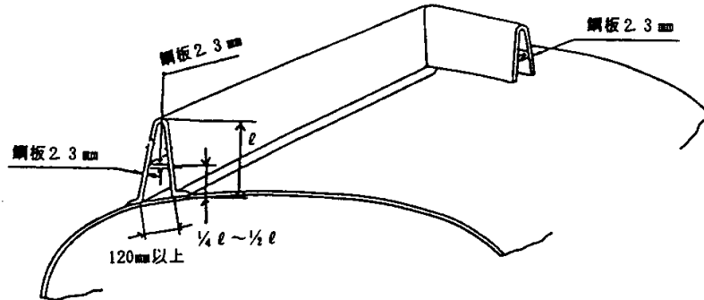
第3-7-23図 防護柵の構造
