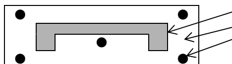
第3-7-21図 1 の締付けボルトに応力集中が発生しない締付け配列方法
