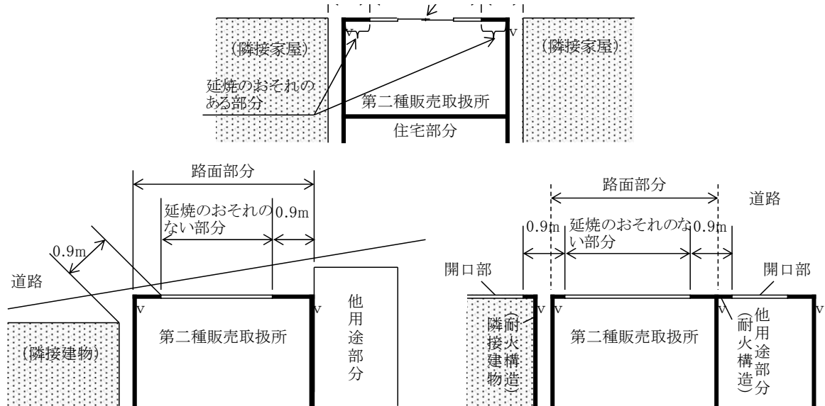
第3-10-4図 延焼のおそれのない部分
