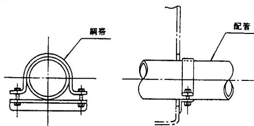
第3-7-31図 吐出口付近の配管の固定方法
