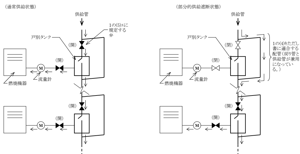
例図4-2 燃料供給系統詳細図（系統例2）
