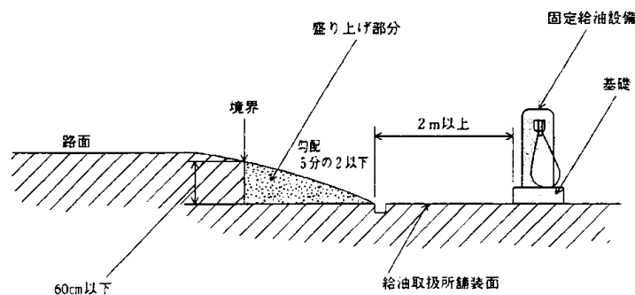
第3-9-9図 道路のかさ上げの場合の例
