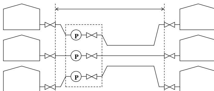
第3-11-6図 移送取扱所の範囲の例（その3）
