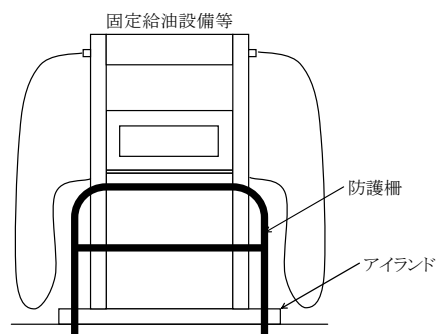
第3-9-29図 衝突防止措置の例
