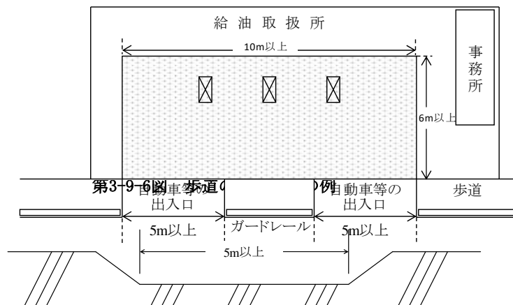
図3-9-5 自動車等の出入口を分割して設置する場合の例※5
