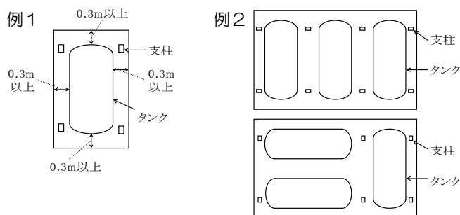
第 3-5-7 図 タンク郡の支柱の例
