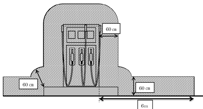
図1 固定給油設備の周囲
