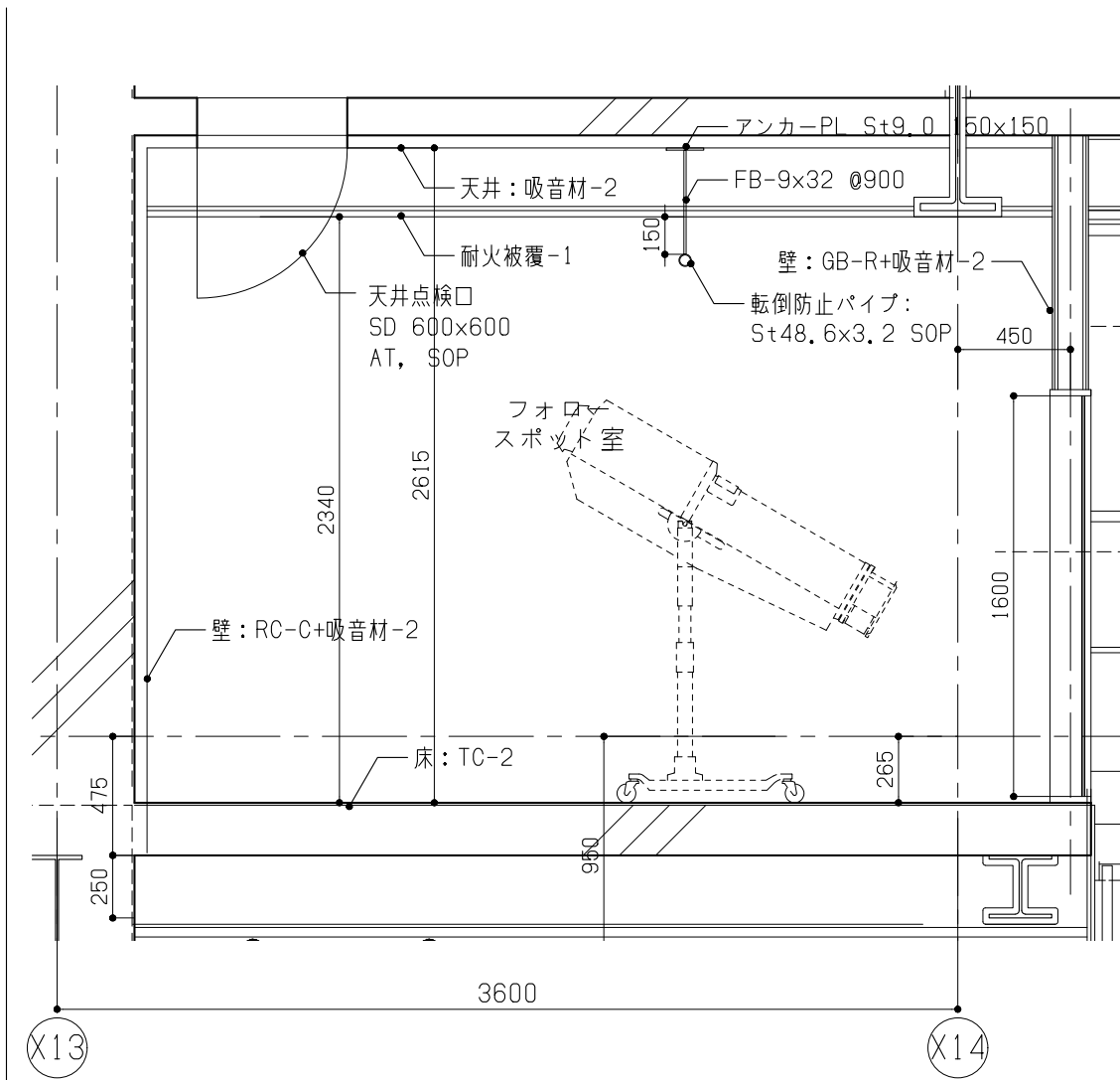
04 フォロースポット室詳細図 A1:1/30 A3:1/60
