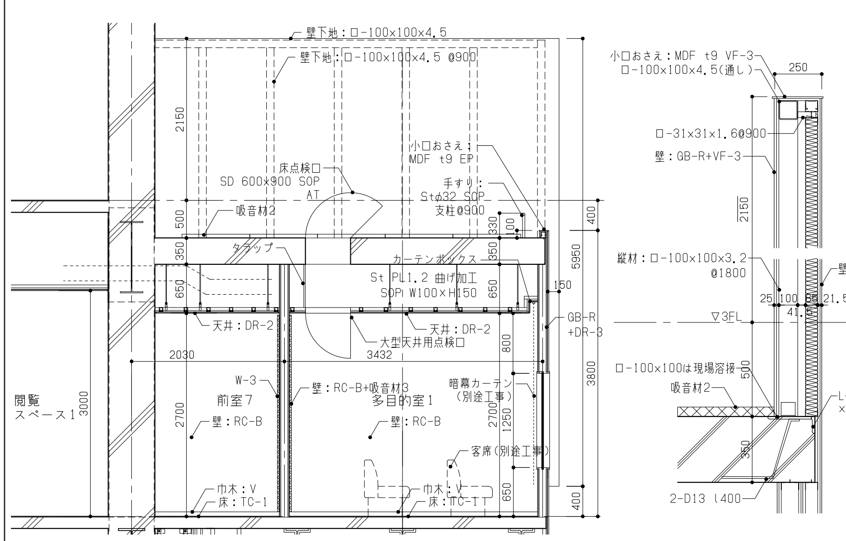
09 客席段床詳細図 A1:1/30 A3:1/60
