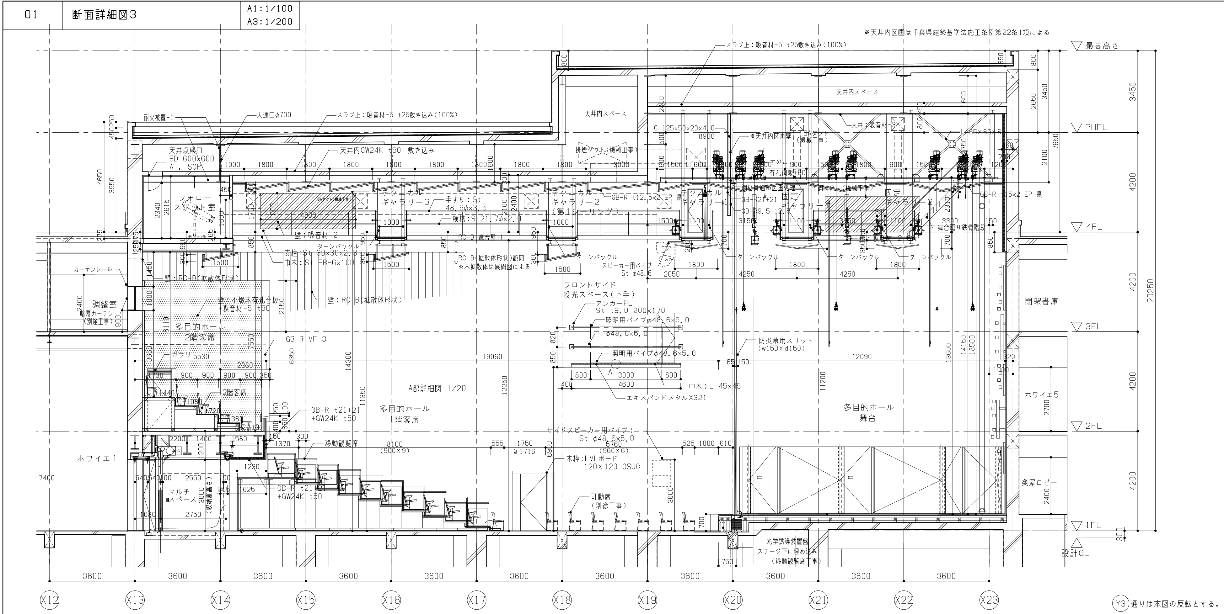
03 多目的室詳細図 A1:1/50, 1/20 A3:1/100, 1/40
