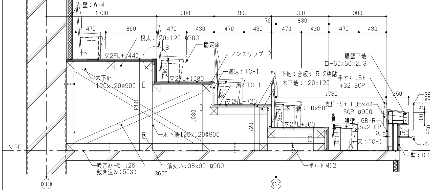
09 客席段床詳細図 A1:1/30 A3:1/60
