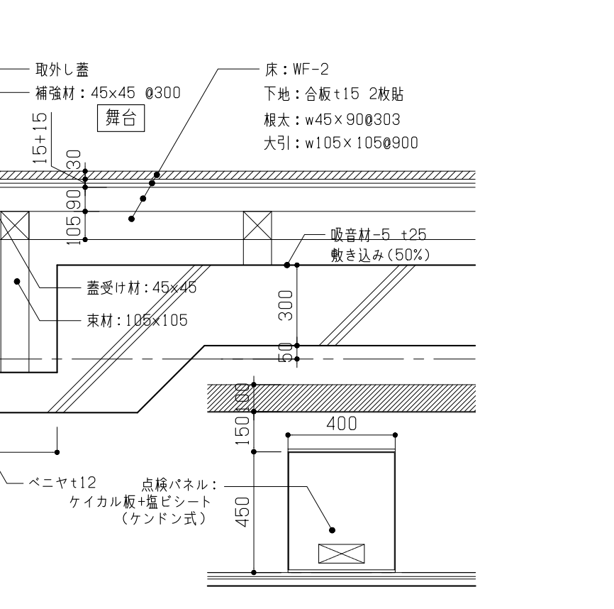
11 舞台床詳細図 A1:1/20 A3:1/40
