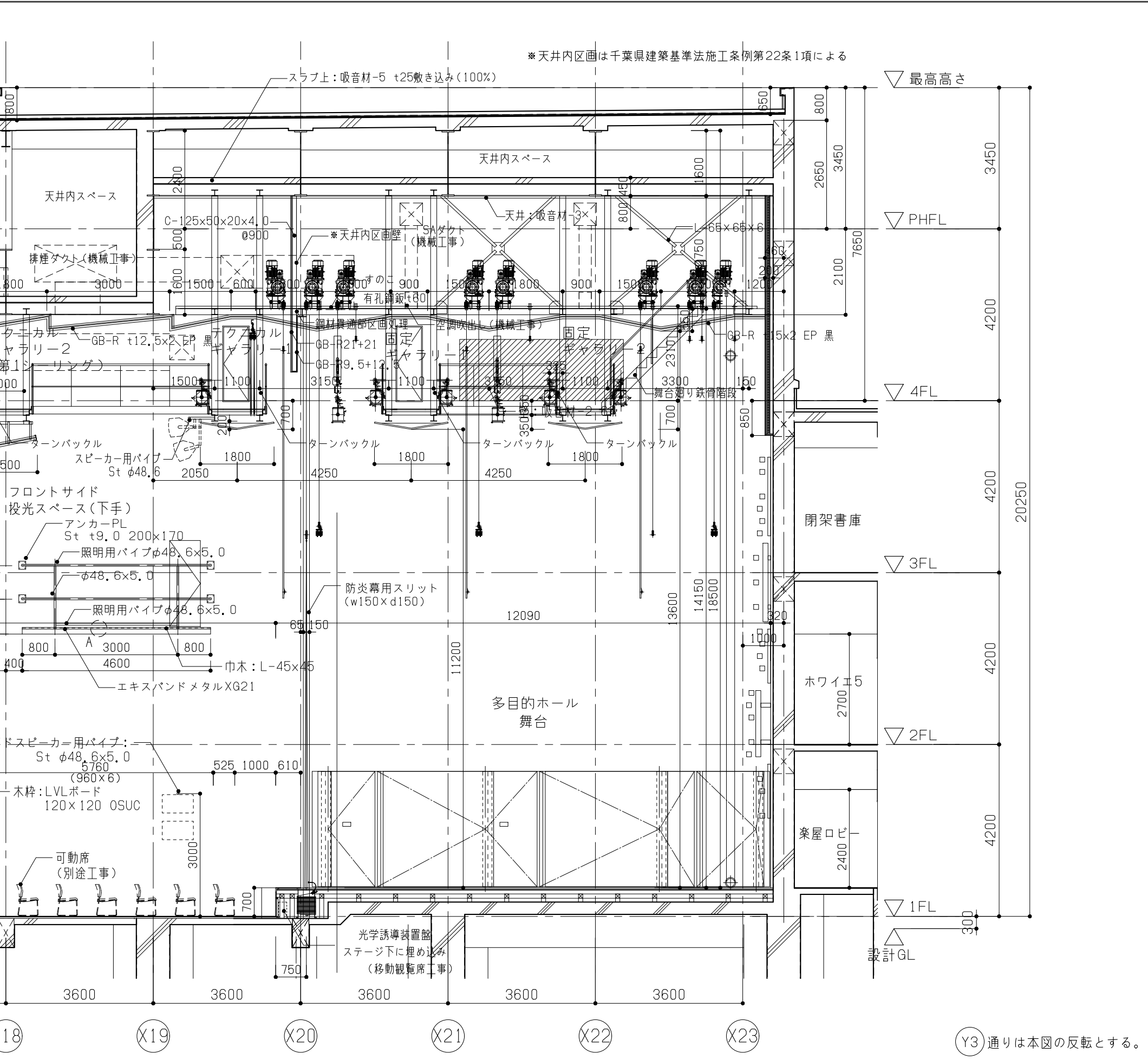
04 フォロースポット室詳細図 A1:1/30 A3:1/60
