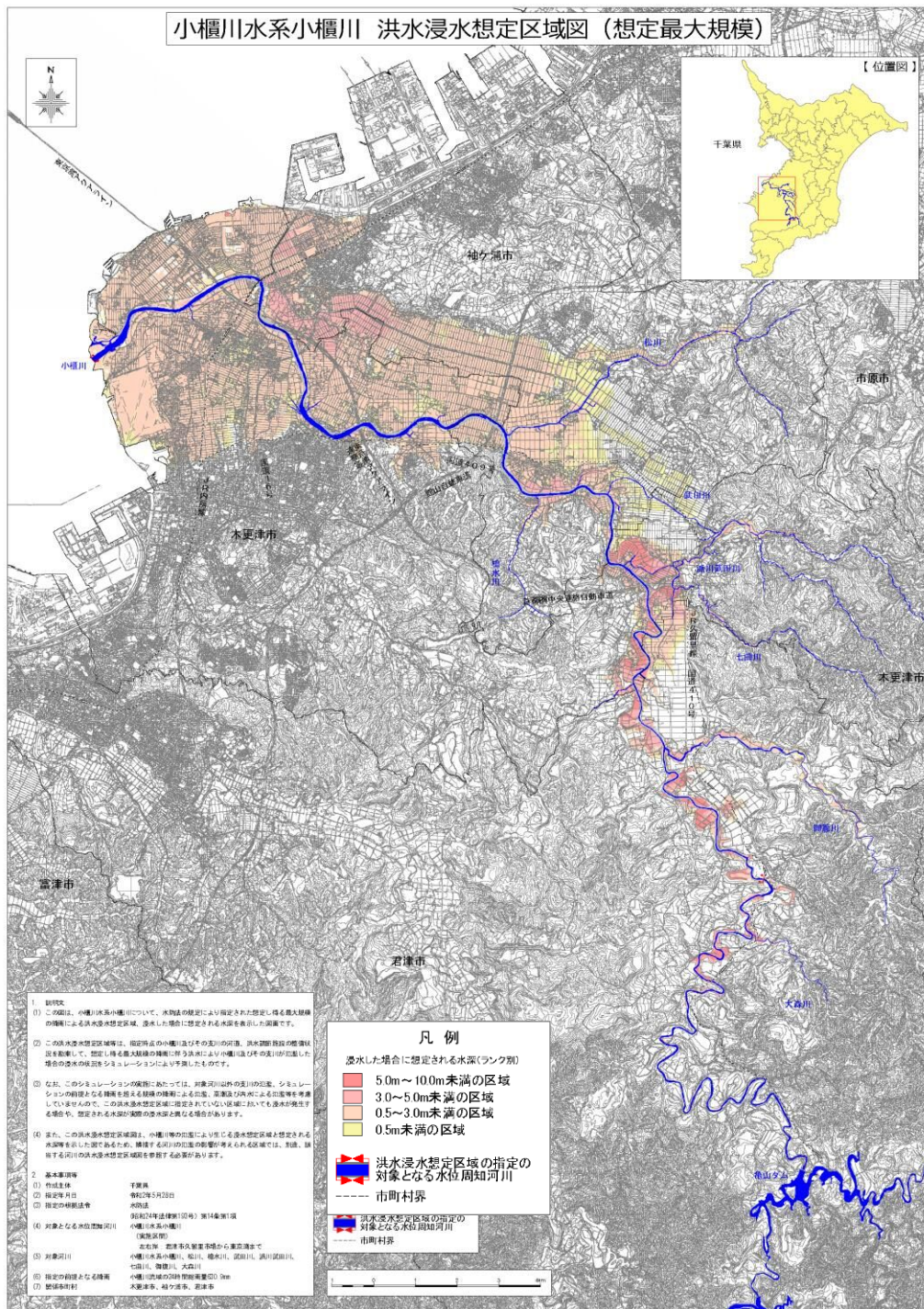
出典：千葉県 小櫃川水系小櫃川洪水浸水想定区域図（想定最大規模）（令和2年5月）
