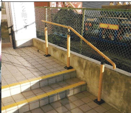
漁協施設(組合事務所)の手摺取付工事 (新木更津市漁業協同組合 岩根支所)
